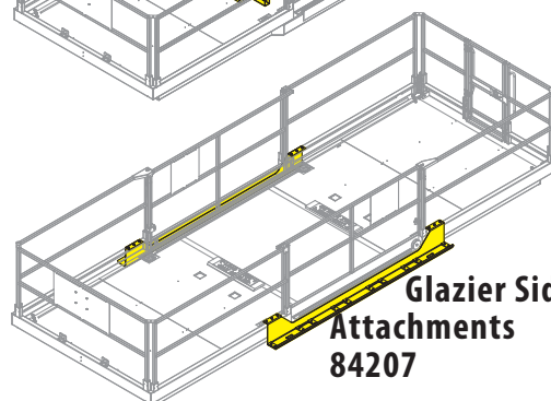
Glazier Rack 84230
